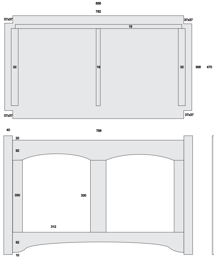
Mortise & Tenon
