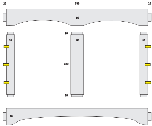
Mortise & Tenon
